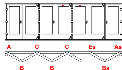
Diagrama 871 (L. marco 4200 ~ 6000mm)
