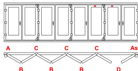
Diagrama 871 (L. marco 4200 ~ 6000mm)
